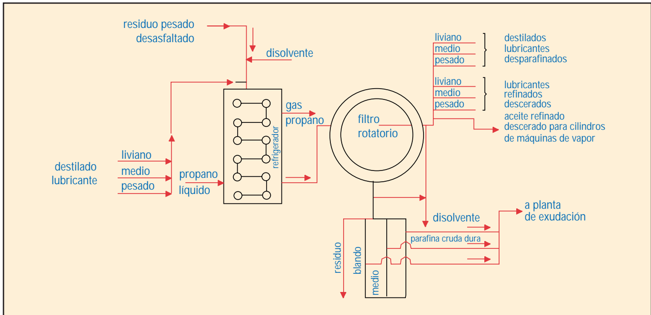
Fig. 6-25. Flujograma del proceso de desceración o desparafinación con disolvente.
