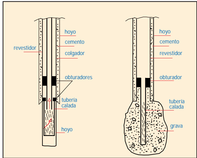
Fig. 4-5. Terminación sencilla con tubería calada. Fig. 4-6. Terminación sencilla y empaque con grava.
