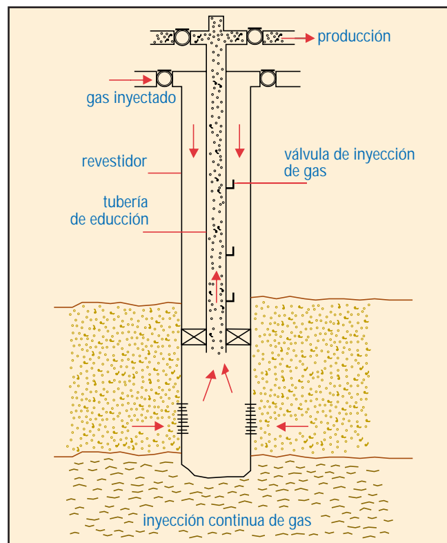
Fig. 4-15. Detalles básicos de una instalación de levantamiento artificial por gas.
