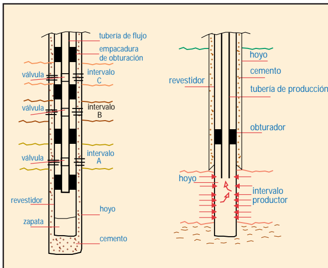
Fig. 4-3. Terminación sencilla de opción múltiple selectiva. Fig. 4-4. Terminación sencilla en hoyo desnudo.
