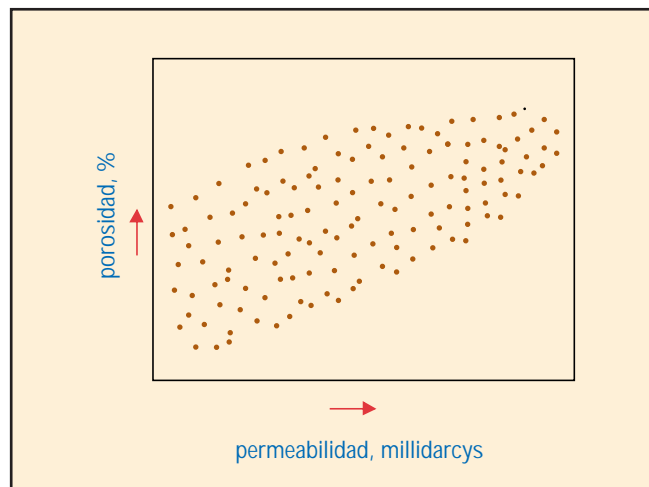
Fig. 4-24. Dispersión de valores de porosidad y permeabilidad.
