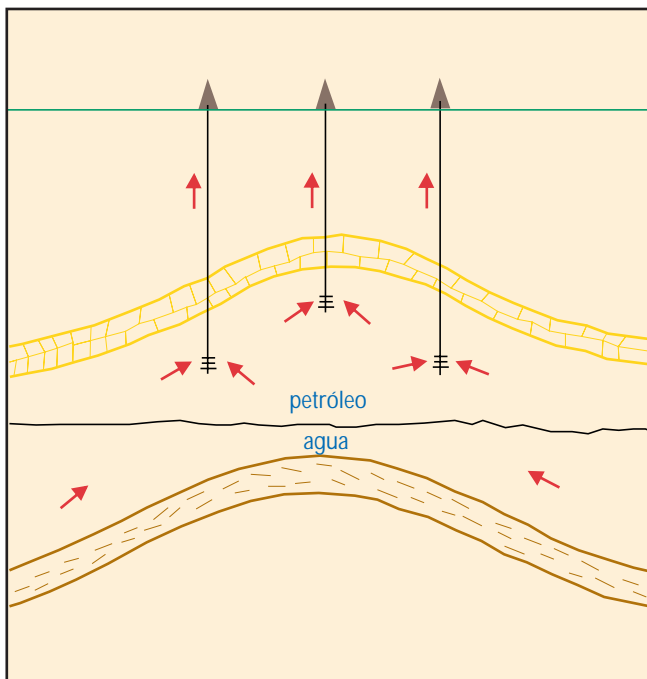
Fig. 4-34. Contacto agua-petróleo en un yacimiento, cuyo mecanismo preponderante de producción será el acuífero, si es lo suficientemente activo.
