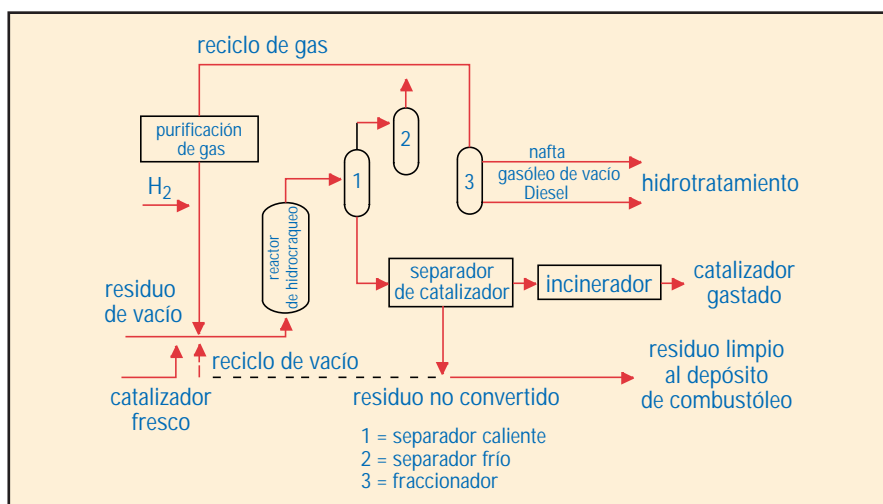
Fig. 11-4. Proceso HDH®.
