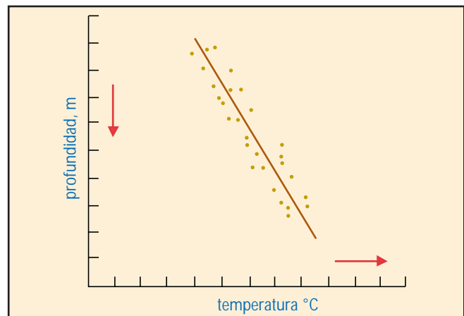
Fig. 4-26. Correlación de valores de profundidad y temperatura en varios pozos.
