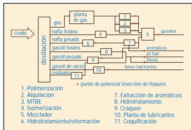
Fig. 11-8. Proceso HYQUIRA™.
