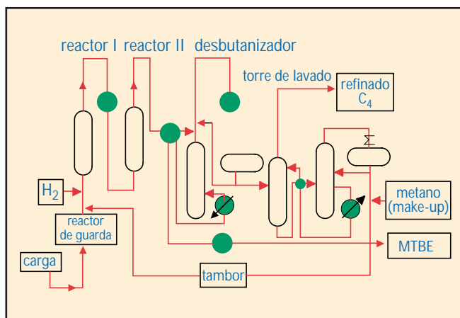
Fig. 11-6. Proceso ETHEROL®.
